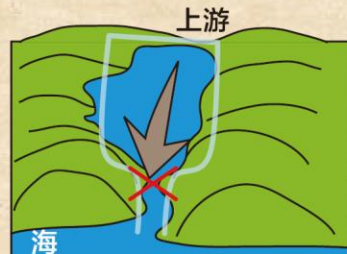
瓶頸狀地形造成泥沙堆積
